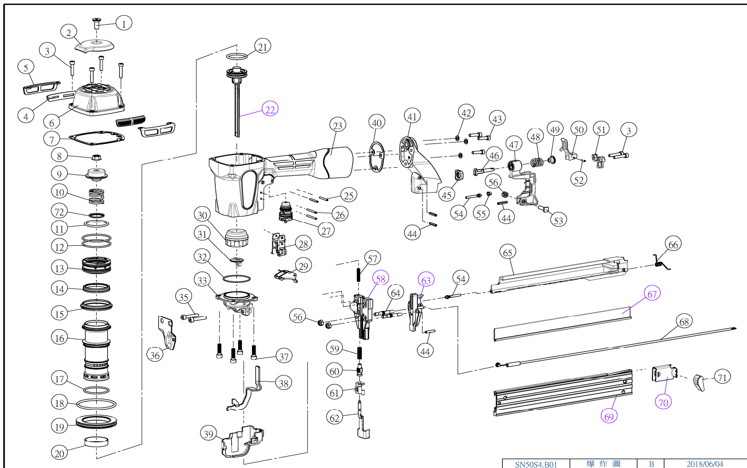
SN50S4.B01 爆炸圖 B 2018/06/04
